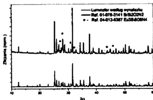
Rys. 1. Dyfrakcja rentgenowska luminoforu według wynalazku. W dolnej części wykresu umieszczono wzorec fazy trójskośnej (PDF-01-076-3141), a strzałkami oznaczono piki odpowiadające fazie \text{Eu}_3\text{Si}_6\text{O}_7\text{N}_4 (PDF-04-013-8367) izomorficznej z fazą \text{Sr}_3\text{Si}_6\text{O}_9\text{N}_4 , która nie posiada swojego wzorca w ogólnie przyjętym zbiorze danych ICDD PDF-4 (edycja 2016).
