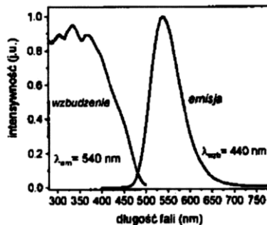
Rys. 2 Widma wzbudzenia otrzymane w maksimum pasma luminescencji dla długości fali 540 nm oraz widma luminescencji otrzymane przy wzbudzeniu długości fali 440 nm.
