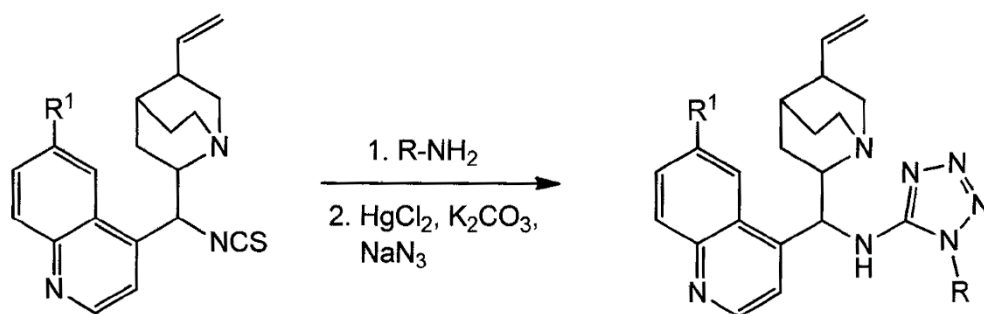
Schemat reakcji
