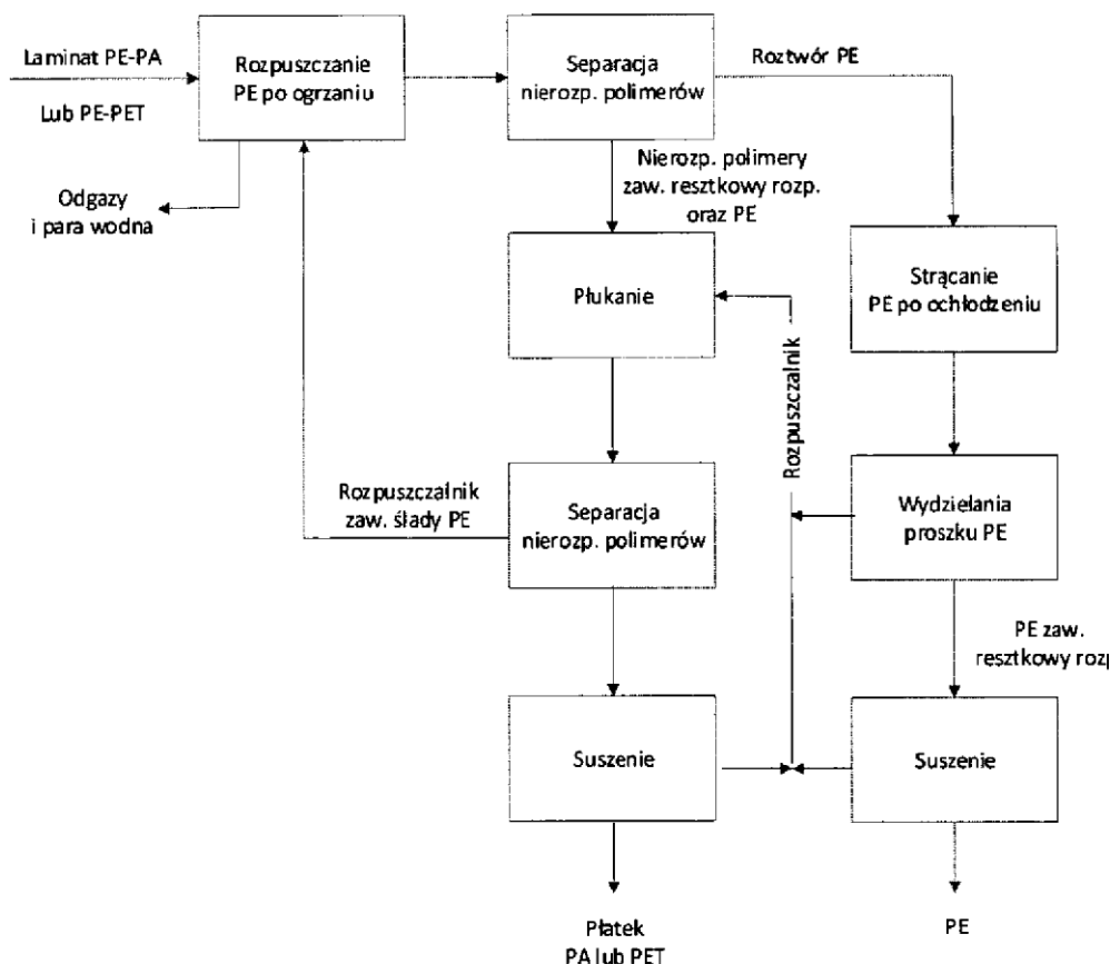
Fig. 1 Schemat blokowy procesu ekstrakcji PE z laminatów PE-PA lub PE-PET wykorzystujący dwa cykle wymywania PE (rozpuszczanie i płukanie)
